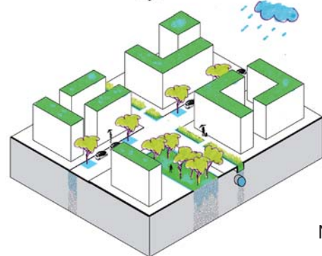
Abb. 09: Stadtquartiere werden stärker durchgrünt, um den Niederschlag wie ein Schwamm aufzusaugen und anschließend zu versickern, zu verdunsten oder gedrosselt abzuleiten.
