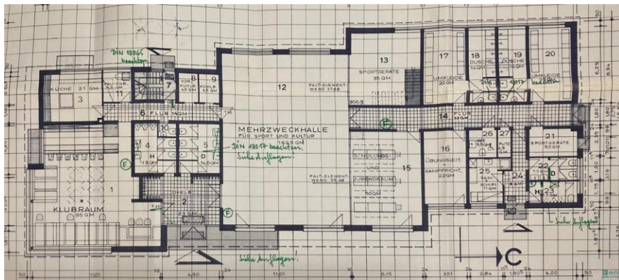
Abbildung 59: Grundriss des Bürgerhauses (GEMEINDE NAHE 1985)
